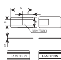
端压片 RU2-ET-A/B
