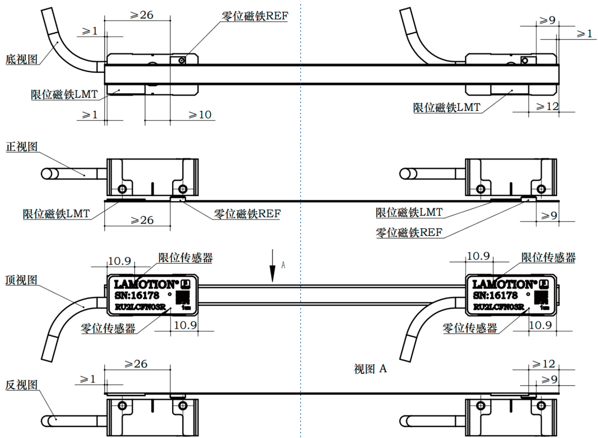
栅尺左端安装零位磁铁
